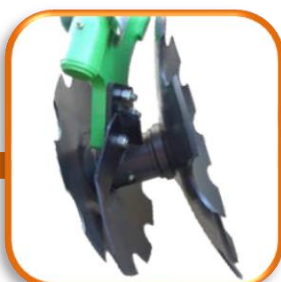
●ダブルディスク φ51cmとφ61cmの異なる 径の組合せが耕起の効率を 向上させます。
