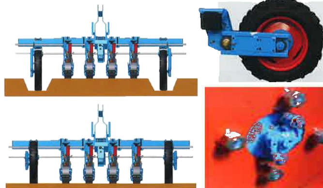
チェーン掛け替え式 / sprocket 交換式
